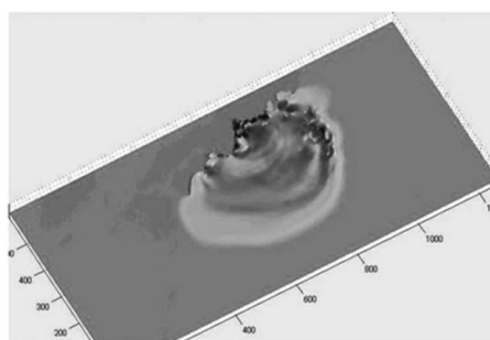
図2 東南海沖地震による津波の発生と伝播のシミュレーションの一例：日本沿岸域への津波来襲までの時間と津波高での予測を数値計算により行う。東南海地震による津波では、東海地方から西国、九州沿岸まで広い範囲での津波の被害が予想されている。
